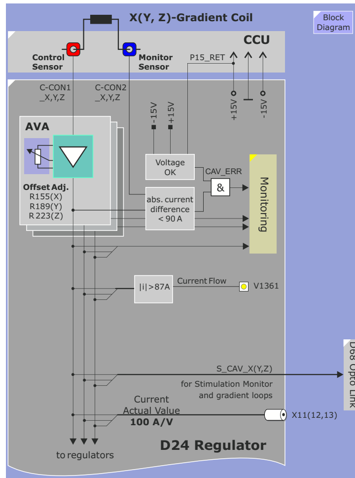
Figure 151 D24 Actual Value Amplifier
