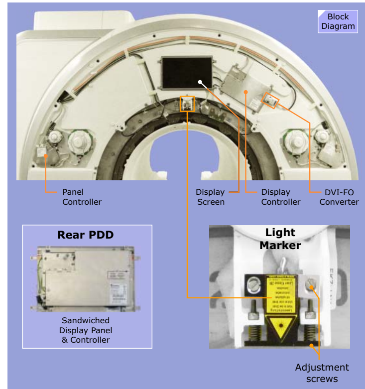
Figure 131 CUI Layout
